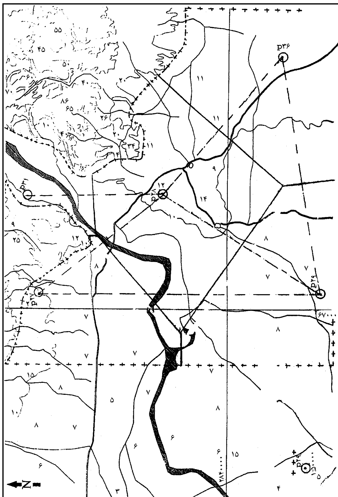
شکل ۱۲-۱ نقشه تیسن بخشی از آبخوان سدیح
