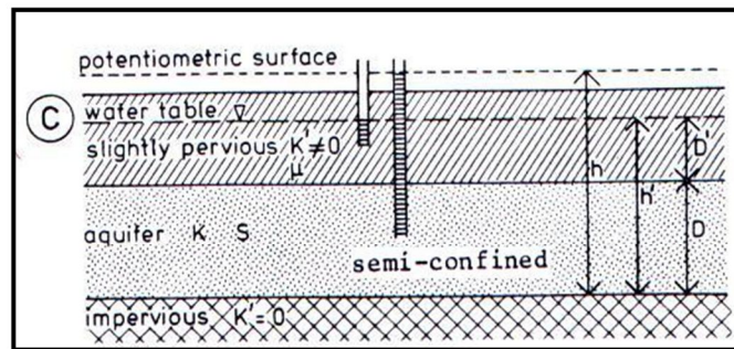
شکل ۱-۴- نمای از یک آبخوان نشتی
