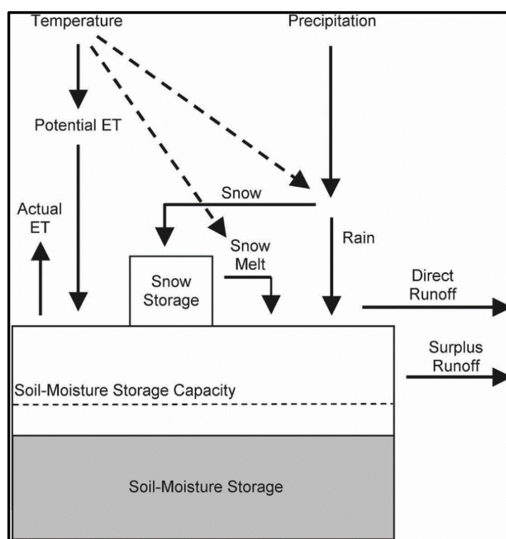
شکل ۴-۱- روند آب در بیلان هیدروکلیماتولوژی
