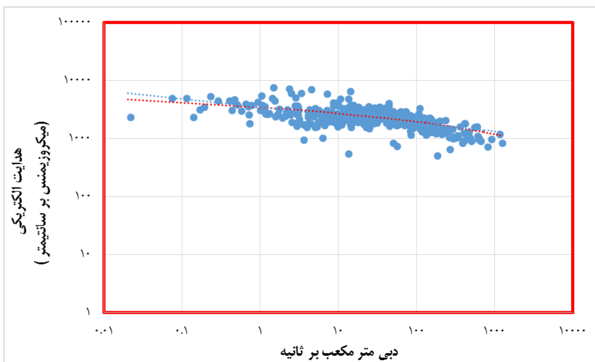
شکل ۹-۱- نمودار دبی-هدایت الکتریکی در ایستگاه هیدرومتری گیلوان
